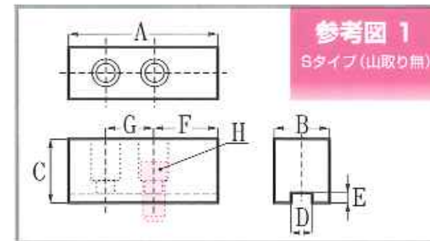
豊和油圧・エアチャック用生爪 価格寸法表
