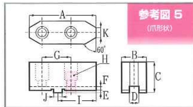
ソールスクロール用生爪 価格寸法表
