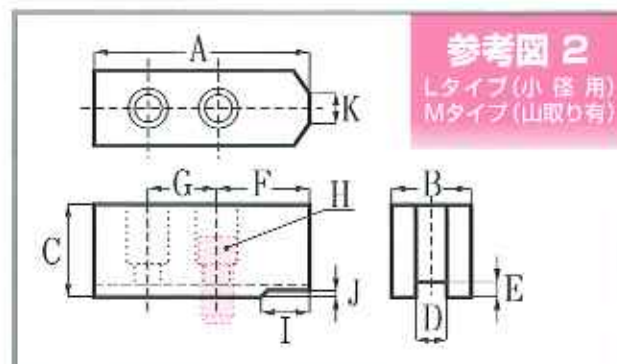
北川油圧・エアーチャック用生爪 価格寸法表
