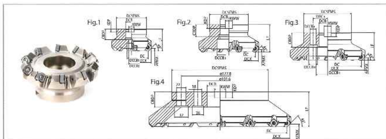
ホルダ寸法
