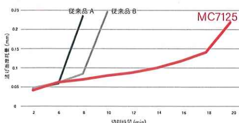
SUS304 断続加工比較
