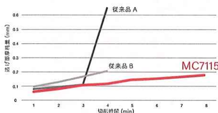
SUS316L 湿式切削加工耐摩耗性試験
